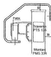
Pièce de guidage N° 1 en inox
